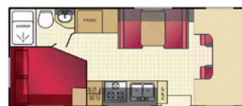
Floorplan C 22 (Grundriss Tag)
